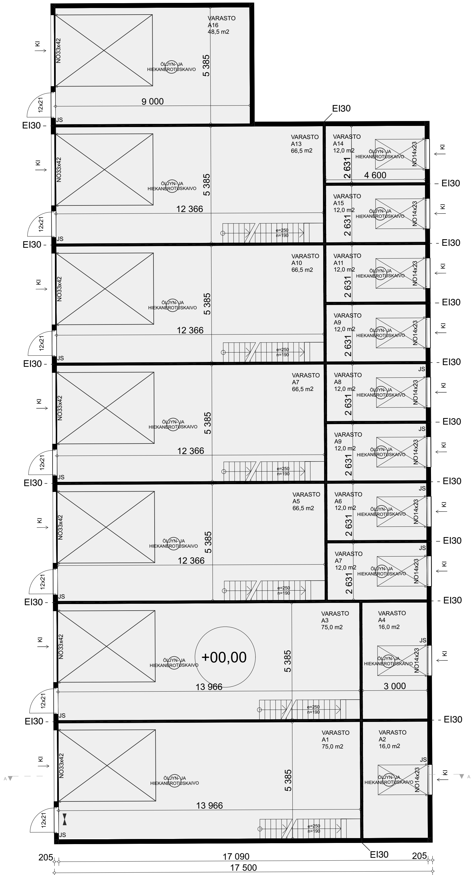
Pohjapiirustus 1.krs 1:100
